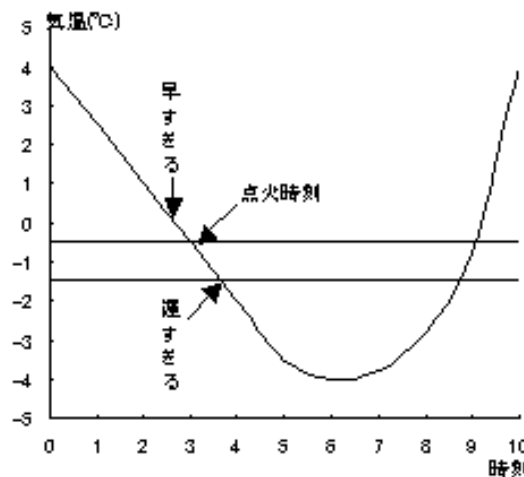
図 4 危険限界温度と点火時刻
