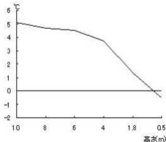
図5 逆転層の出現状況(小松1994)
