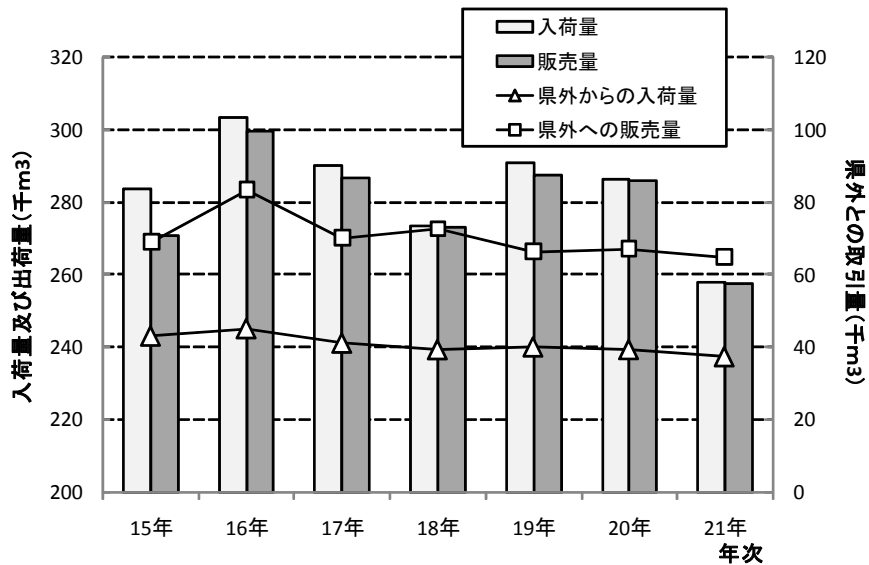
図-3 素材の市場入出荷量の推移
