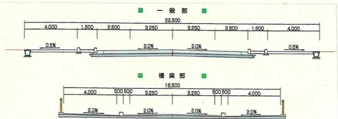
標準横断面図
